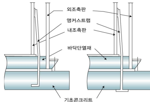
그림 2.2.3.7 평저형 저장탱크의 앵커스트립 설치방법
