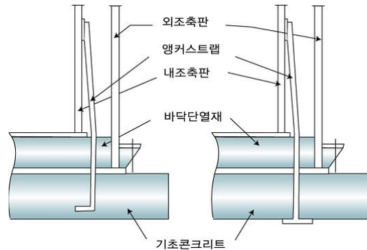
그림 2.2.3.7 평저형 저장탱크의 앵커스트립 설치방법
