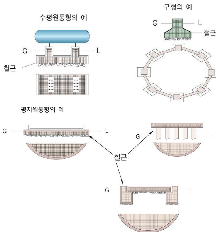
그림 2.2.2.3 저장탱크의 수평기초면
