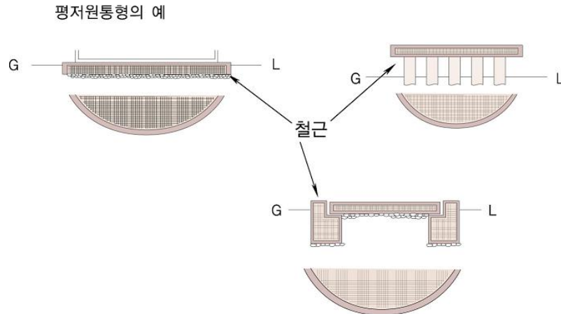
그림 2.2.2.3 저장탱크의 수평기초면
