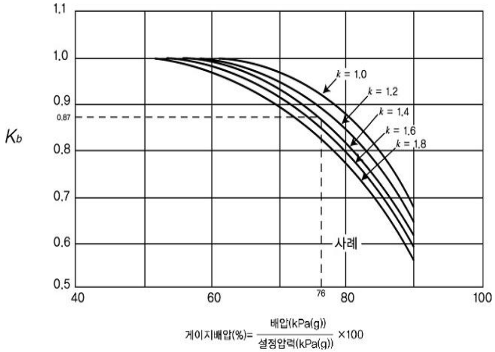
그림 2.6.1.4③ Conventional 안전밸브 배압조정계수
