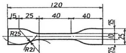
그림 B6②. 신장영구늘음률 시험용 시편 예
