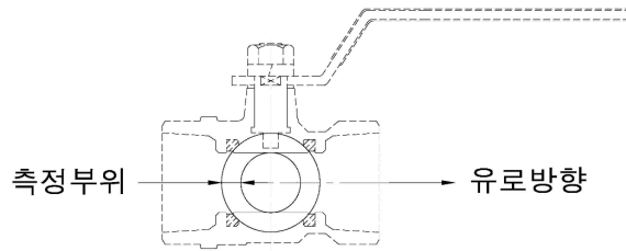
그림 3.3.1 볼 중심부 두께 측정부
