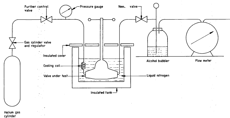
그림 3.8.1.2.3 초저온밸브 기밀시험(예시)
