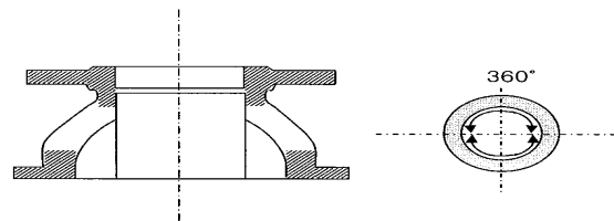
< 플랜지 밸브 >
