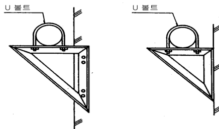
(a) 브라켓지지
