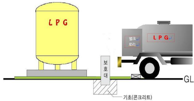
그림 2.3.3.4(6) 보호대 설치방법
