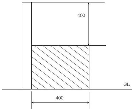
그림 2.9.2.2.3 보조벽의 높이
