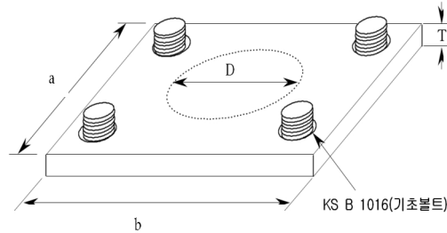
그림 2.3.3.2(5-3-2) 강판제 보호대의 받침대 설치 방법
