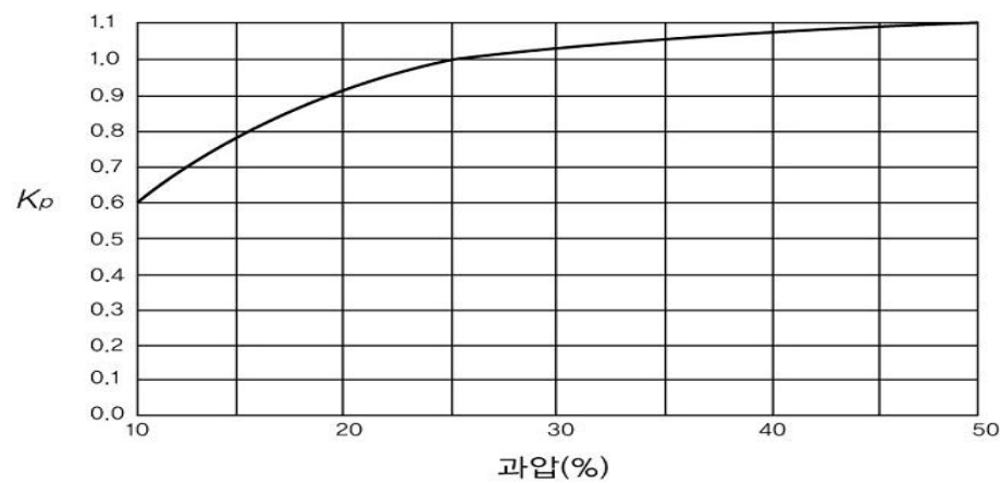
그림 2.8.1.4.1(2)⑧ 과압보정계수
