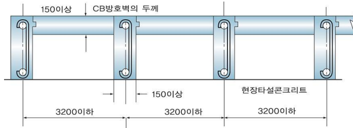
그림 2.9.2.2.2 보조벽의 배치
