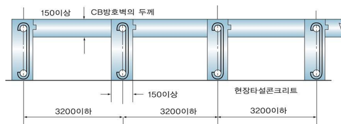
그림 2.9.2.2.2 보조벽의 배치
