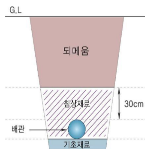
그림 2.5.7.5.5 배관의 매설방법
