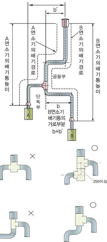
그림 2.7.1.3.1(3) 복합배기통 설치 예
