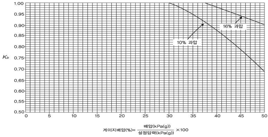
그림 2.8.1.4.1(2)② 벨린스 벨로우즈형 안전밸브 배압보정계수
