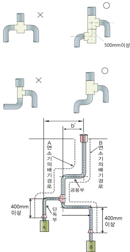
그림 2.7.1.3.2 복합 배기통의 설치 예
