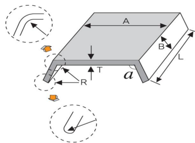
그림 2.5.7.5.3 보호판의 치수
