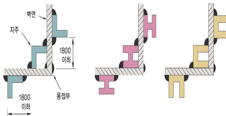
그림 2.9.2.3.4 지주의 설치방법
