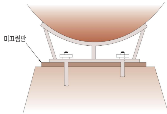
그림 2.2.3.5 미끄럼판의 설치방법
