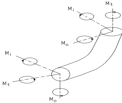
그림 1. 곡관부에 작용하는 모멘트
