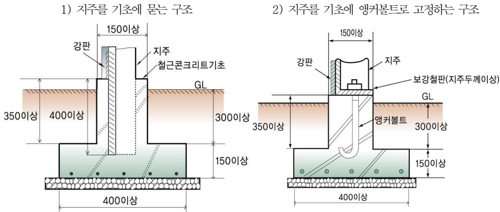
그림 2.8.2.3.6 강판제 방호벽의 고정방법 예
