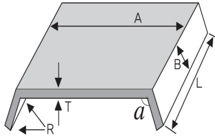
그림 2.5.8.2.3 보호관의 치수 측정
