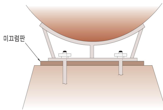
그림 2.2.3.5 미끄럼판의 설치방법
