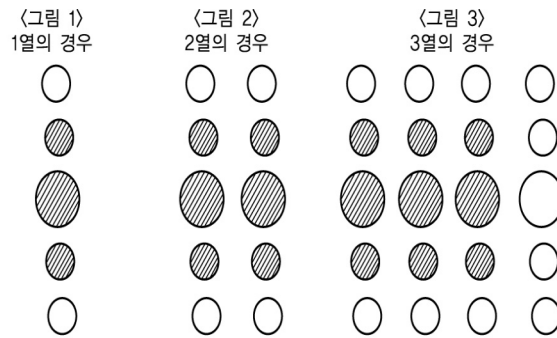
주) 사선 친 부분의 저장탱크가 대상표면적이 됨.
