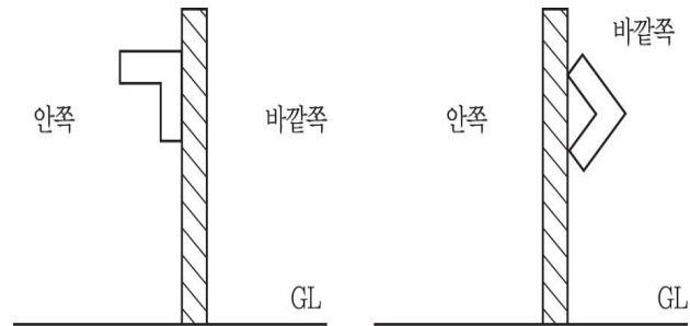
그림 2.8.2.3.2 강관제방호벽의 앵글강 보강
