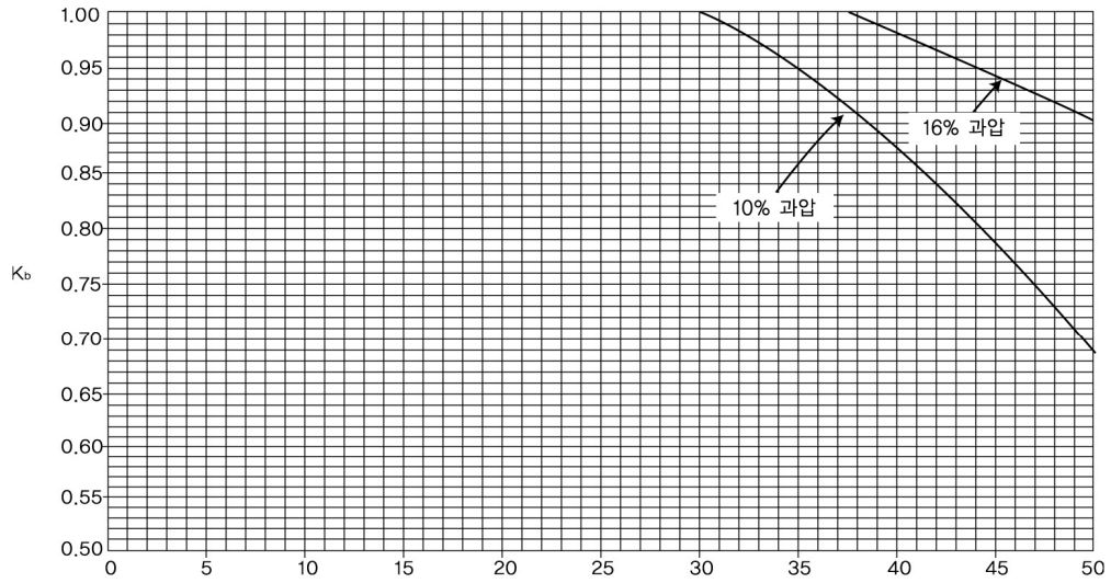
그림 2.6.1.4② 밸런스 벨로우즈형 안전밸브 배압보정계
