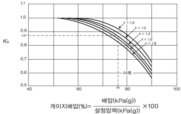
그림 2.6.1.4(2)③ Conventional 안전밸브 배압조정계수
