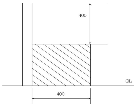
그림 2.7.2.2.4 보조벽의 높이
