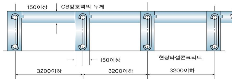
그림 2.7.2.2.3 보조벽의 배치
