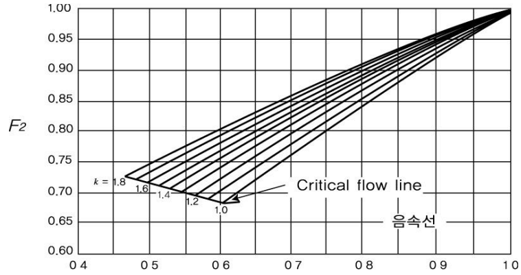
그림 2.6.1.4(2)⑤ 이음속계수
