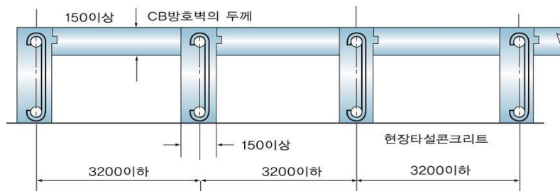
그림 2.7.2.2.3 보조벽의 배치
