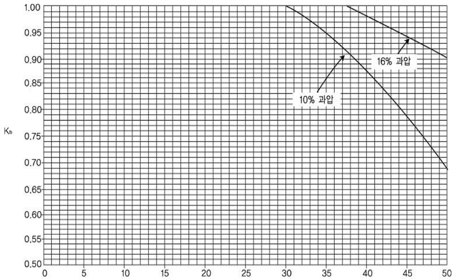
그림 2.6.1.4① 열용량비 k=C_p/C_v
