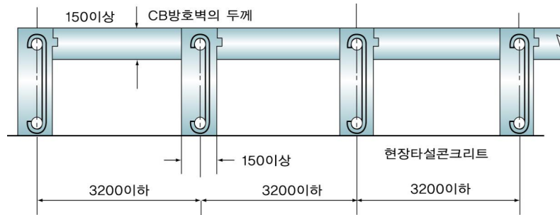
그림 2.7.2.2.2 보조벽의 배치
