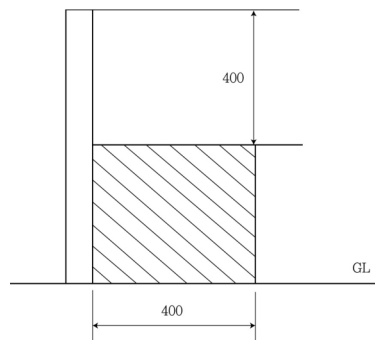
그림 2.7.2.2.3 보조벽의 높이
