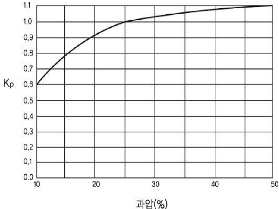
그림 2.6.1.4⑧ 과압보정계수
