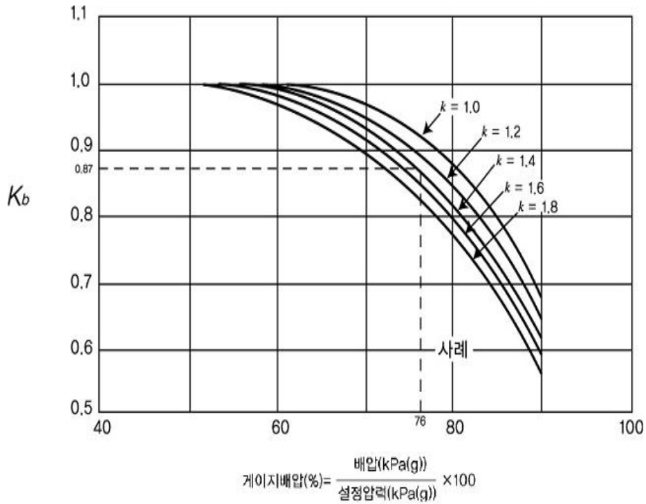
그림 2.6.1.4③ Conventional 안전밸브 배압조정계수
