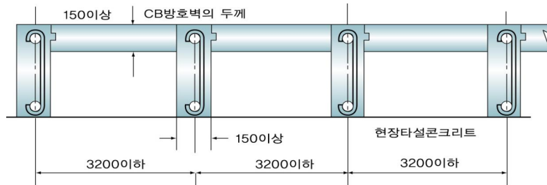
그림 2.7.2.2.2 보조벽의 배치
