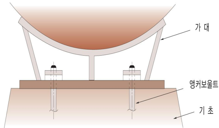
그림 2.2.3.4 앵커보울트의 고정방법
