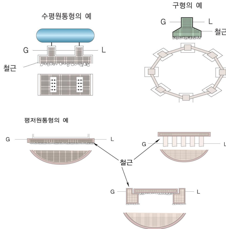
그림 2.2.2.3 저장탱크의 수평기초면
