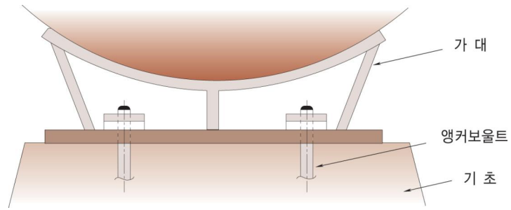
그림 2.2.3.4 앵커보울트의 고정방법
