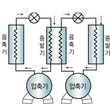
(3) 이원냉동설비
