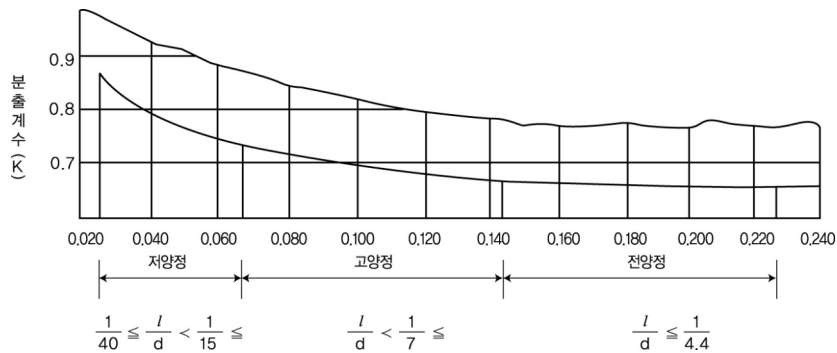
그림 2.6.1.2 분출계수
