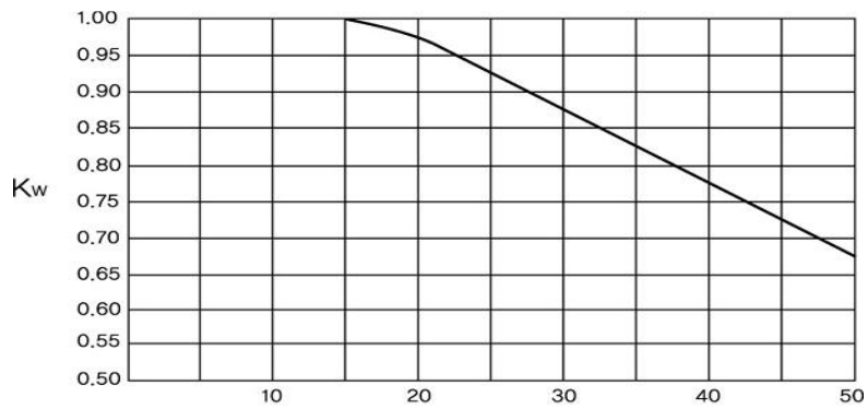
그림 2.6.1.4⑤ 아음속계수
