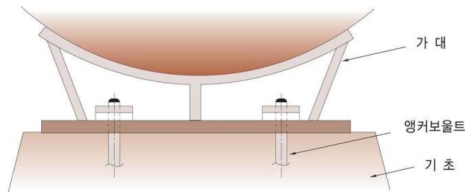
그림 2.2.3.4 앵커보울트의 고정방법
