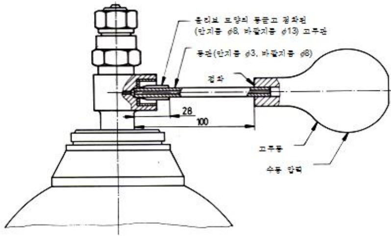
그림 B.1 약한 용기 밸브를 확인하는 장비
