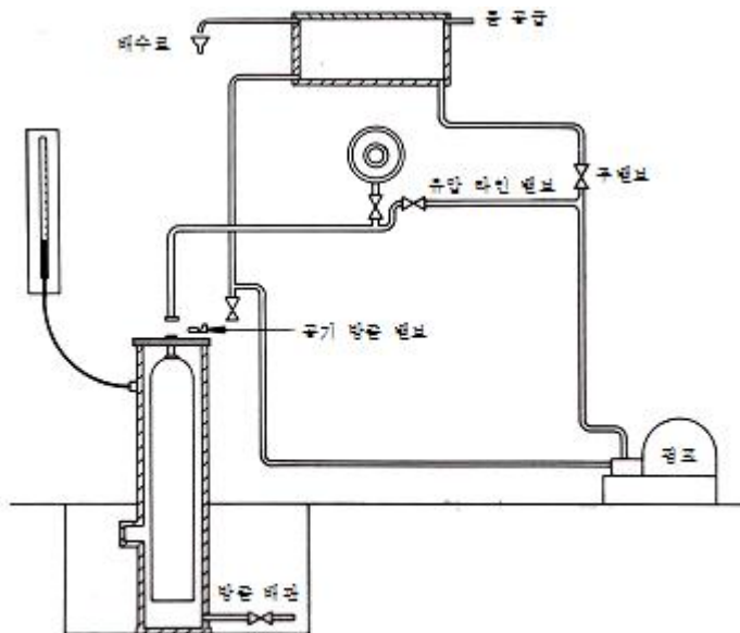
그림 F.2 워터 재킷 누피 평가 시험-고정 유액 방법
