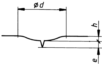
부속서 3 그림 3 굽힌 흠 또는 찌힌 흠을 포함하는 우그러짐
