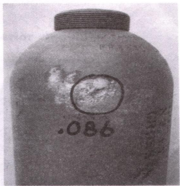
그림 C.2 면 부식
