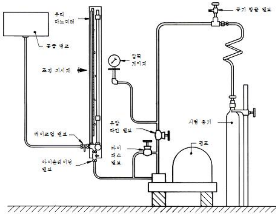
그림 F.3 워터 재킷이 없는 제적 평창 시험
