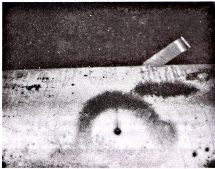
그림 C.1 단독 피트
