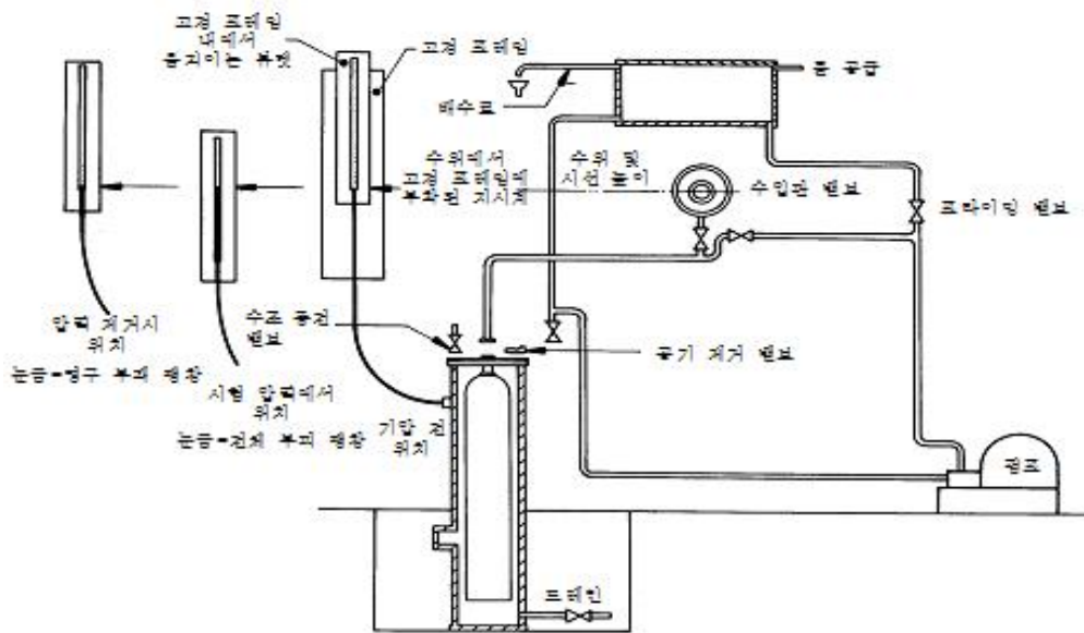
부속서 5 그림 1 수조식 부피 팽창 시험-필연류법
