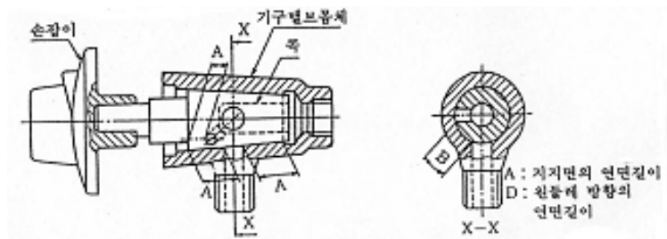
그림 3.2.20.3 콕 구조의 기구 밸브
