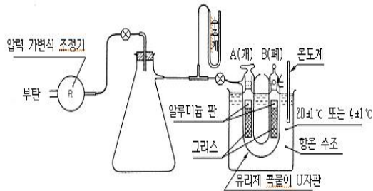
그림 C2. 내가스성 시험을 위한 시험장치
