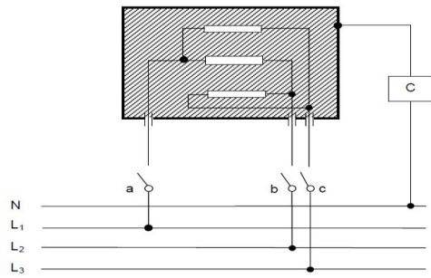
그림 C20②. 누설전류 시험회로 (3상4선)
