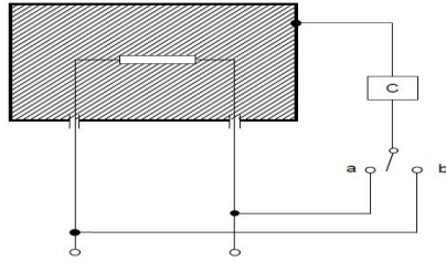
그림 C20①. 누설전류 시험회로 (단상2선)
