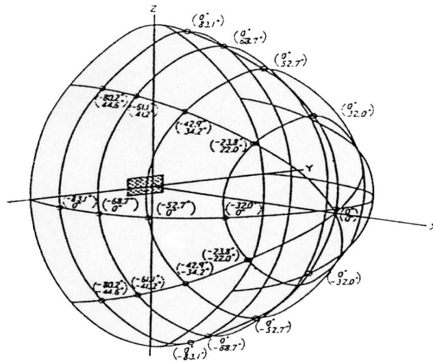
그림 C6 . 방사각도의 측정
