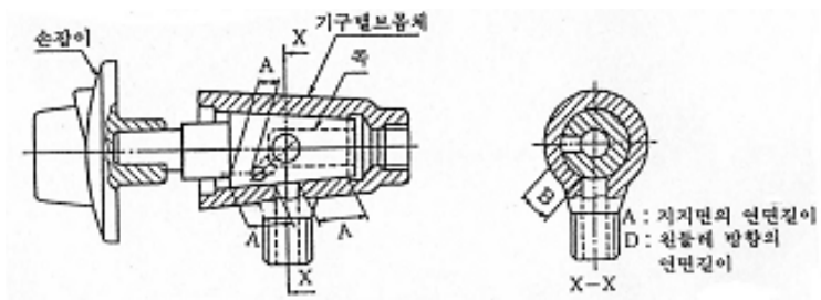
그림 3.2.24.3 콕 구조의 기구 밸브
