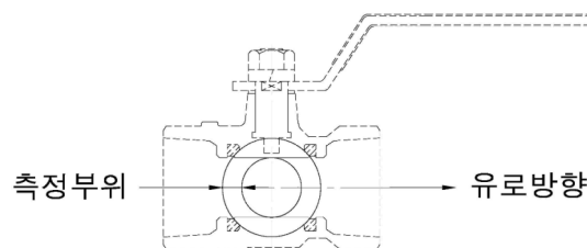
그림 3.3.1 볼 중심부 두께 측정부
