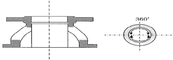
< 플랜지 밸브 >
