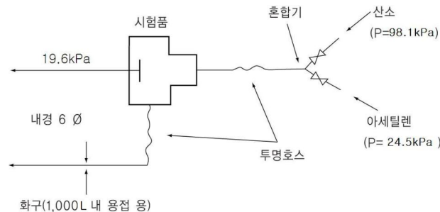
그림 3.8.1.4 역화방지시험 방법
