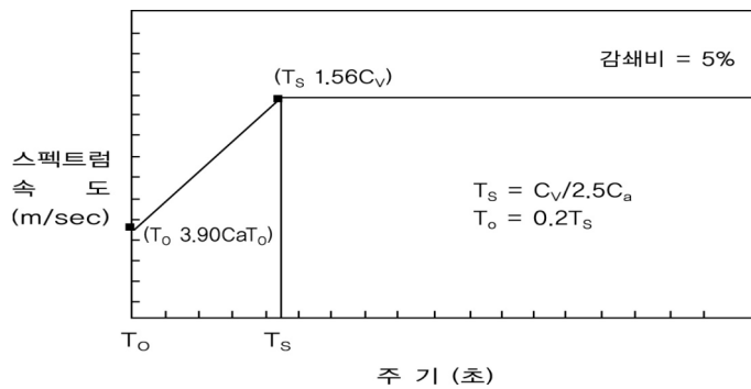
그림 2.4.6.1.1 표준설계응답스펙트럼
