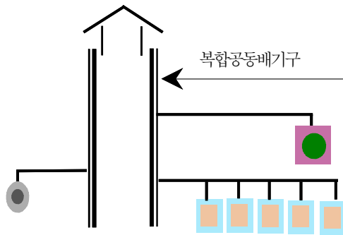
그림 2.7.1.3.2② 복합공동배기구 시공 예
