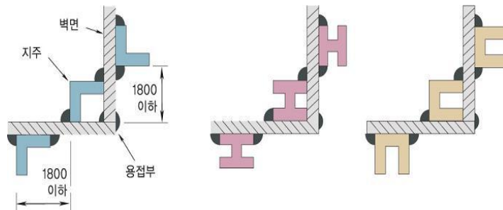
그림 2.9.2.3.4 지주의 설치방법
