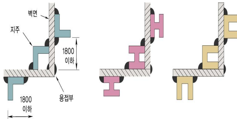
그림 2.9.2.3.4 지주의 설치방법
