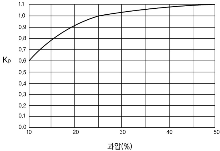
그림 2.8.1.4.2③ 과압보정계수
