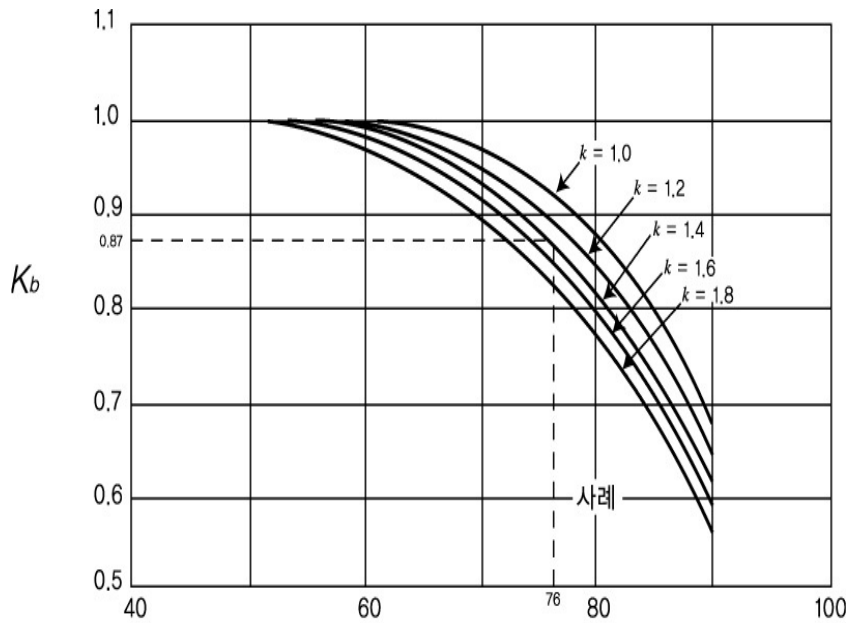
그림 2.7.1.2② 평형벨로우즈형 과압안전장치 배압보정계수
