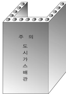
그림 2.5.8.3(3) 철근콘크리트 방호조치
