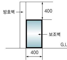
그림 2.8.2.2.3 보조벽의 높이
