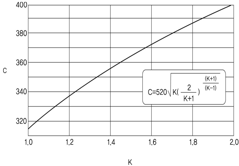
그림 2.7.1.4.1① 열용량비 k=C_p/C_v
