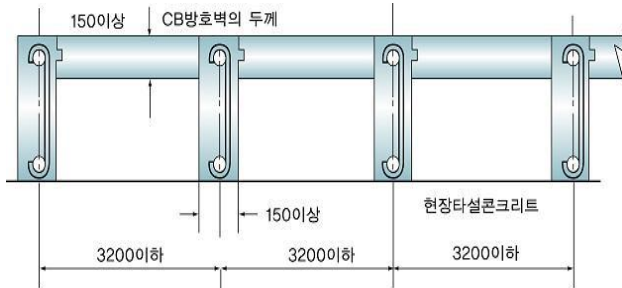
그림 2.8.2.2.2 보조벽의 배치
