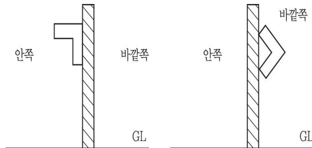
그림 2.8.2.3.2 강판제방호벽의 앵글강 보강
