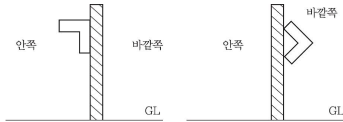
그림 2.7.2.3.2 강판제방호벽의 앵글강 보강
