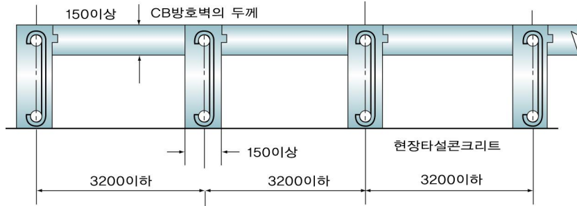
그림 2.7.2.2 보조벽의 배치
