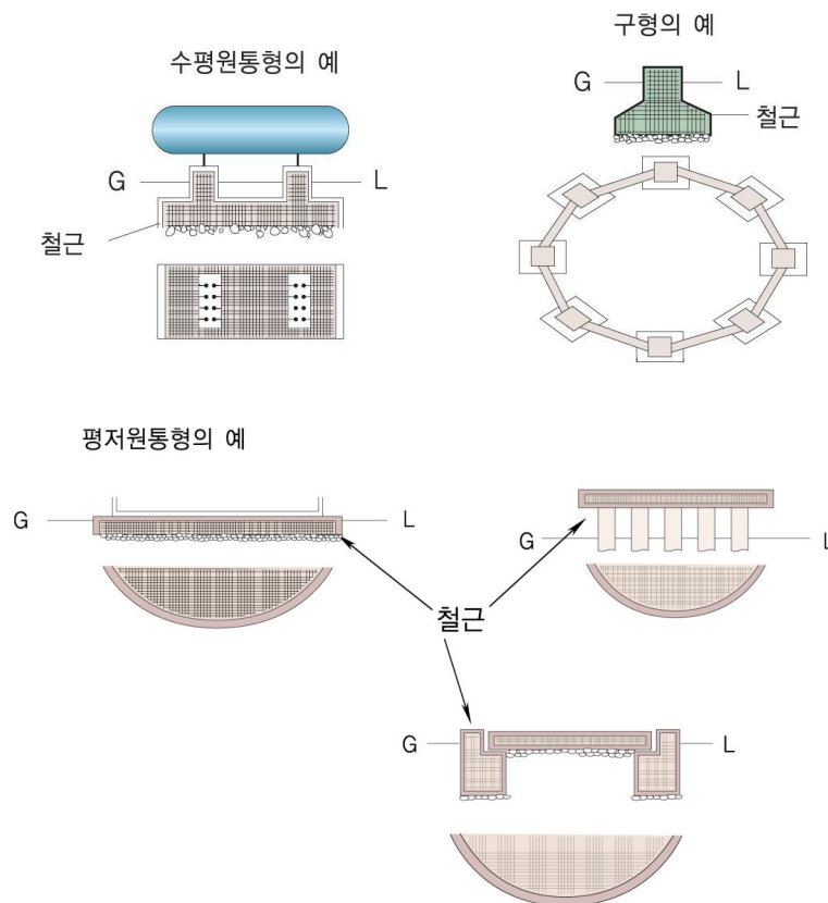
그림 2.2.2.3 저장탱크의 수평기초면
