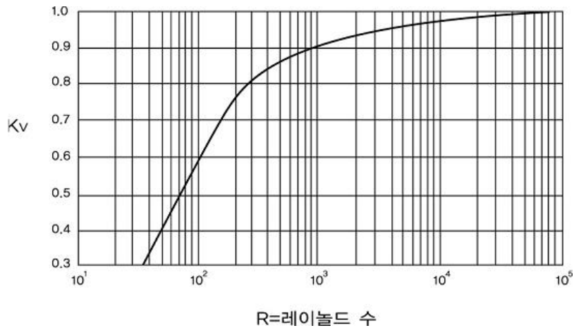
R=레이놀드 수 그림 2.6.1.4⑦ 점도로 인한 용량보정계수
