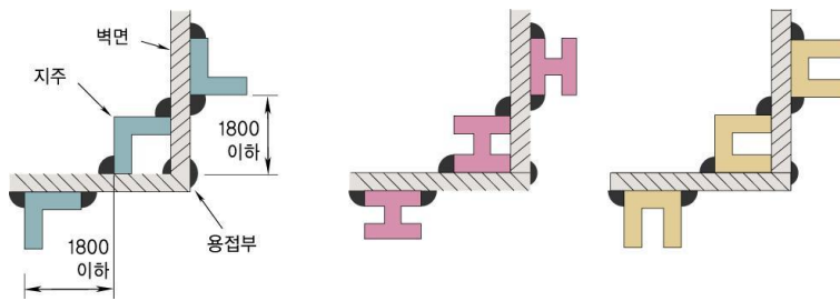
그림 2.7.2.3.4 지주의 설치방법
