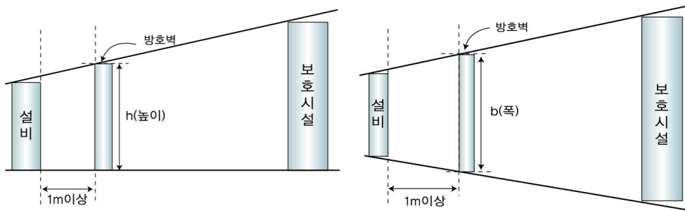
그림 2.7.2.1.1① 방호벽 설치 예(측면도)
