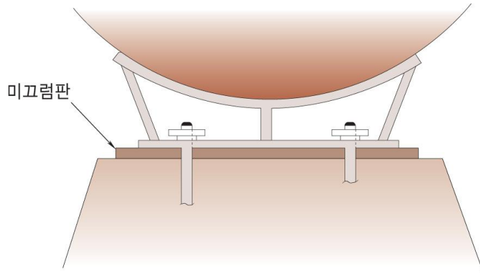
그림 2.2.3.5.3 미끄럼판의 설치방법
