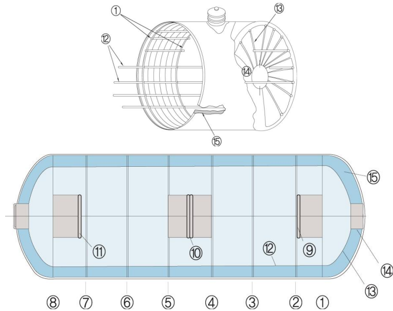
전 체 조 립 도
