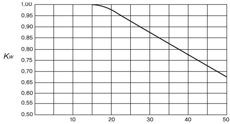
그림 2.6.1.4(2)⑤ 아음속계수
