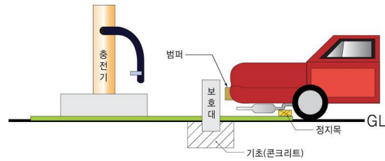
그림 2.4.4.2.2(2) 보호대 설치방법
