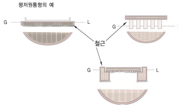
그림 2.2.2.4 저장탱크의 수평기초면
