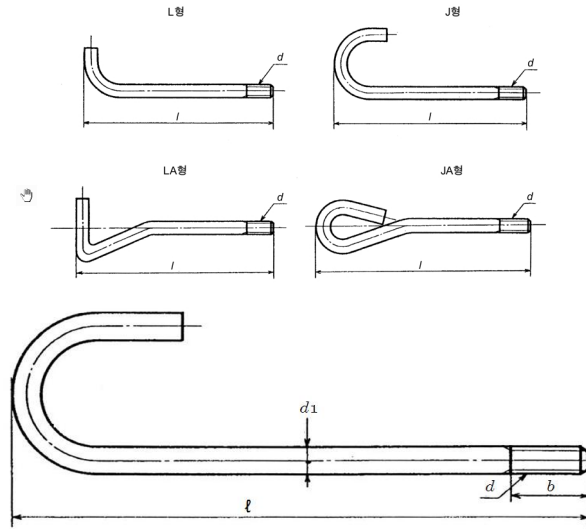
그림 2.2.3.3.1 앵커볼트의 모양
