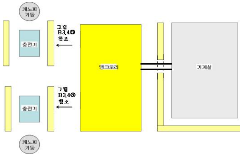
그림 B3.4② 보호대 설치 평면도 예시
