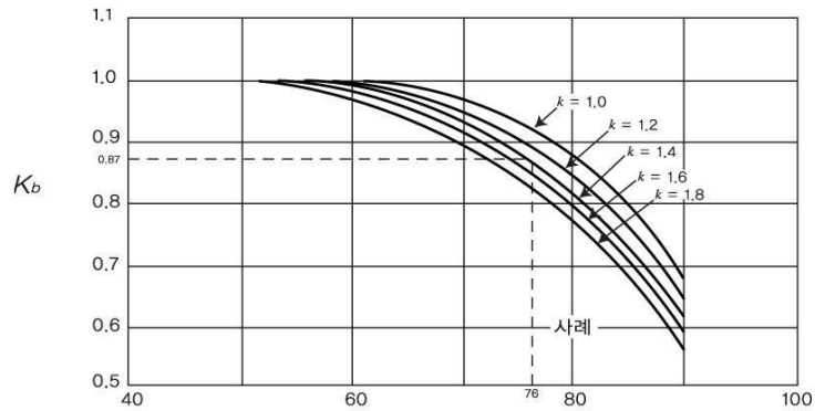
그림 2.6.1.4(2)② 밸런스 벨로우즈형 안전밸브 배압보정계수
