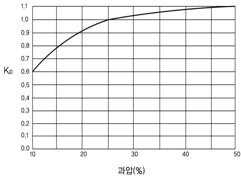
그림 2.6.1.4.2③ 과압보정계수
