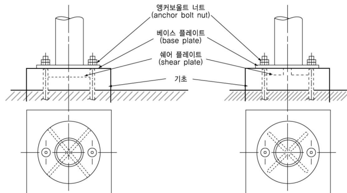
그림 2.2.3.6 구형저장탱크 지주와 기초에 앵커보울트 체결방법
