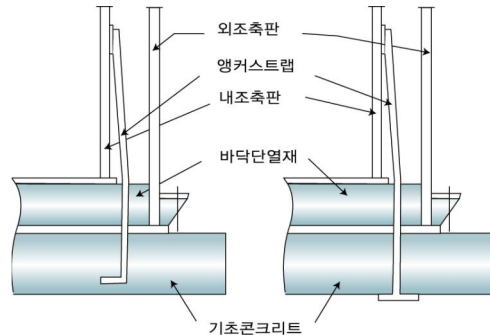
그림 2.2.3.7 평저형 저장탱크의 앵커스트립 설치방법
