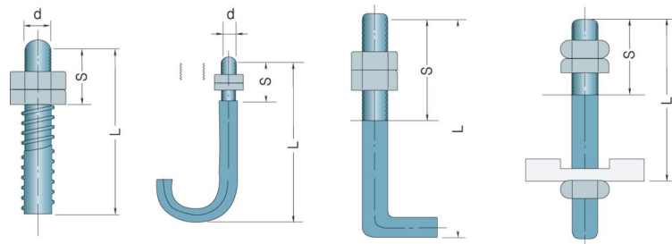
그림 2.2.3.3 앵커보울트의 치수표시
