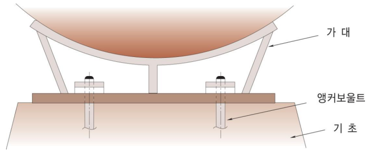
그림 2.2.3.4 앵커보울트의 고정방법
