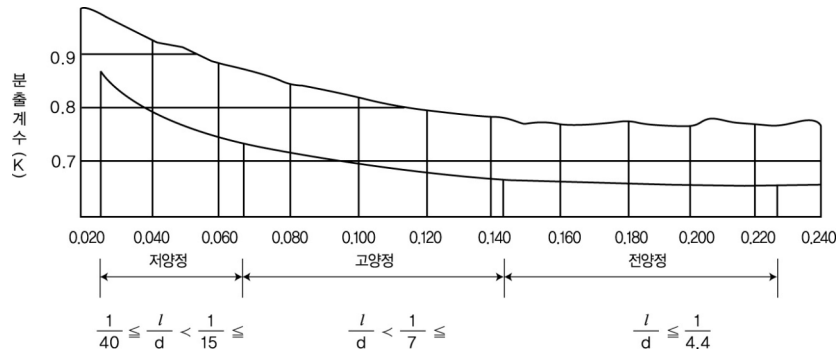
그림 2.6.1.2 분출계수
