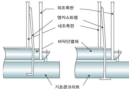
그림 2.2.3.7 평저형 저장탱크의 앵커스트랩 설치방법
