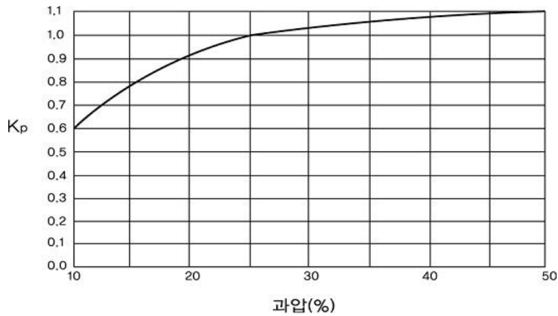
그림 2.6.1.4⑧ 과압보정계수
