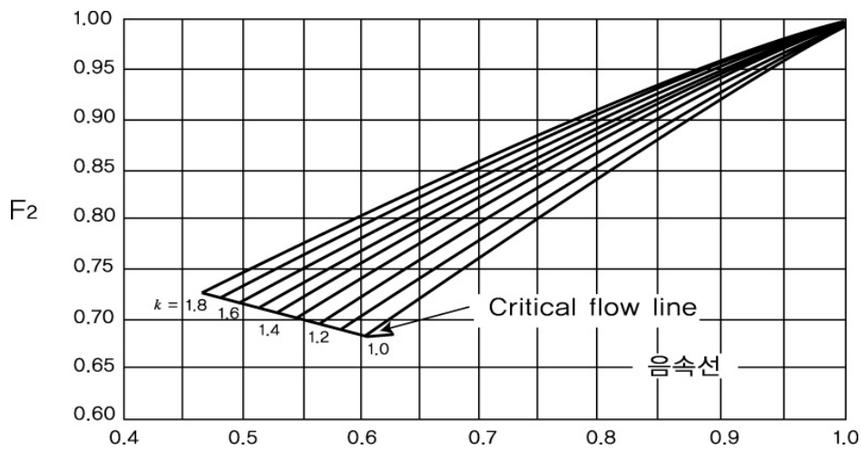
그림 2.6.1.4⑤ 아음속계수
