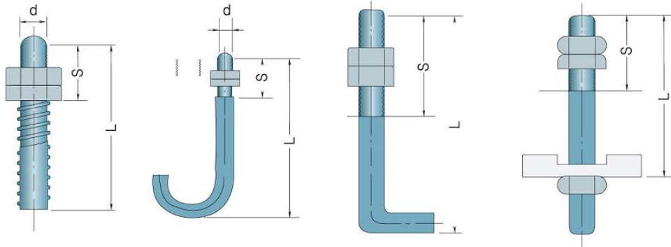
그림 2.2.3.3 앵커보울트의 치수표시
