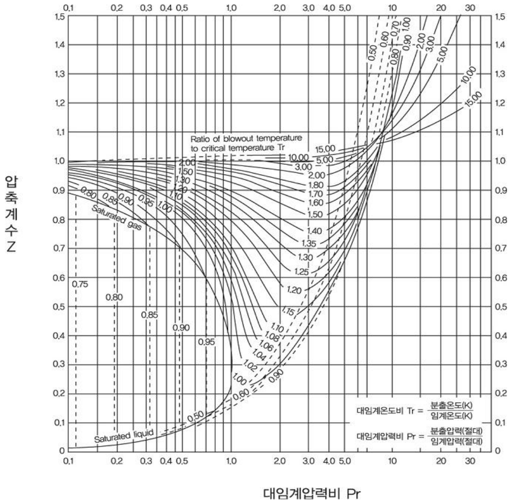
그림 2.6.1.4④ 압축계수
