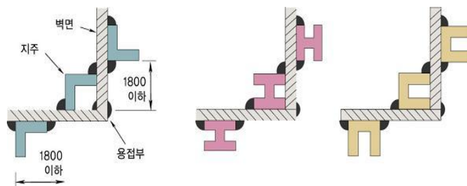
그림 2.7.2.3.4 지주의 설치방법
