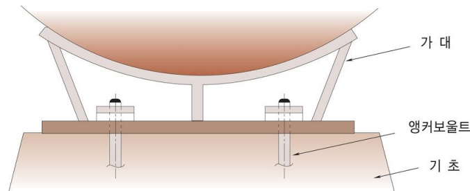
그림 2.2.3.4 앵커보울트의 고정방법
