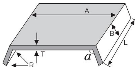
그림 2.5.7.2.3(4) 보호관의 치수 측정
