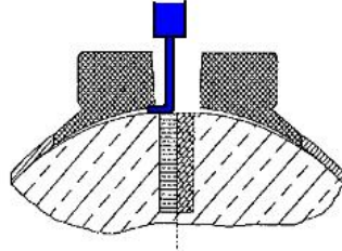
그림 5.2.1.2.2 틈새부 간격 측정 방법
