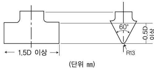
그림 4.4.2.1(2)③ 압력시험용 강제빼기
