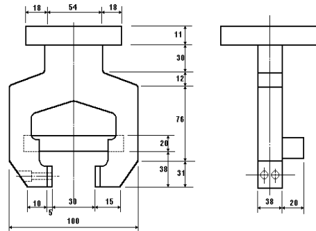
그림 3.11.2.2 벨브 부 착 치 구(예시)
