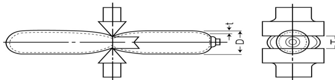
그림 4.4.2.1(2)③ 압력시험용 강제빼기
