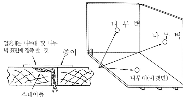
그림 C7. 나무대 및 나무벽 표면 온도 측정 장치
