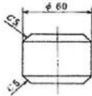
그림 3.4.2.6.1 낙하체의 형상
