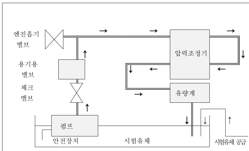
그림 B2. 액중펌프를 부착한 시험장치
