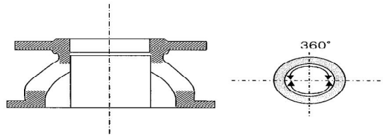
그림 3.8.2.2.1 방사선투과시험 부위(예시)
